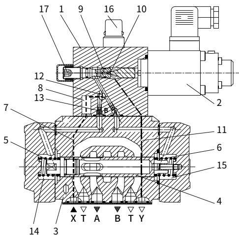
3DREM10P-L6X/...G24K4V 型
